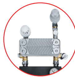
Warmtewisselaar met RTL en thermostaatventiel
